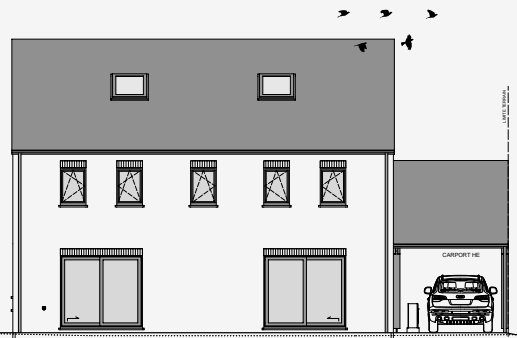
Façade arrière
