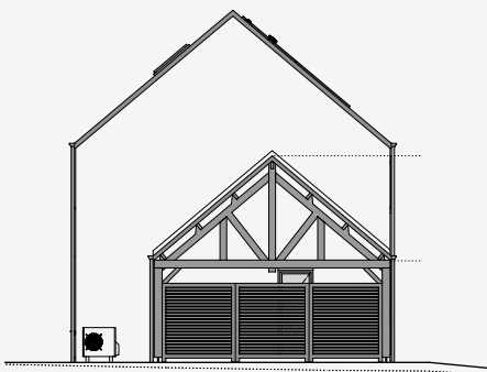
Pignon gauche
